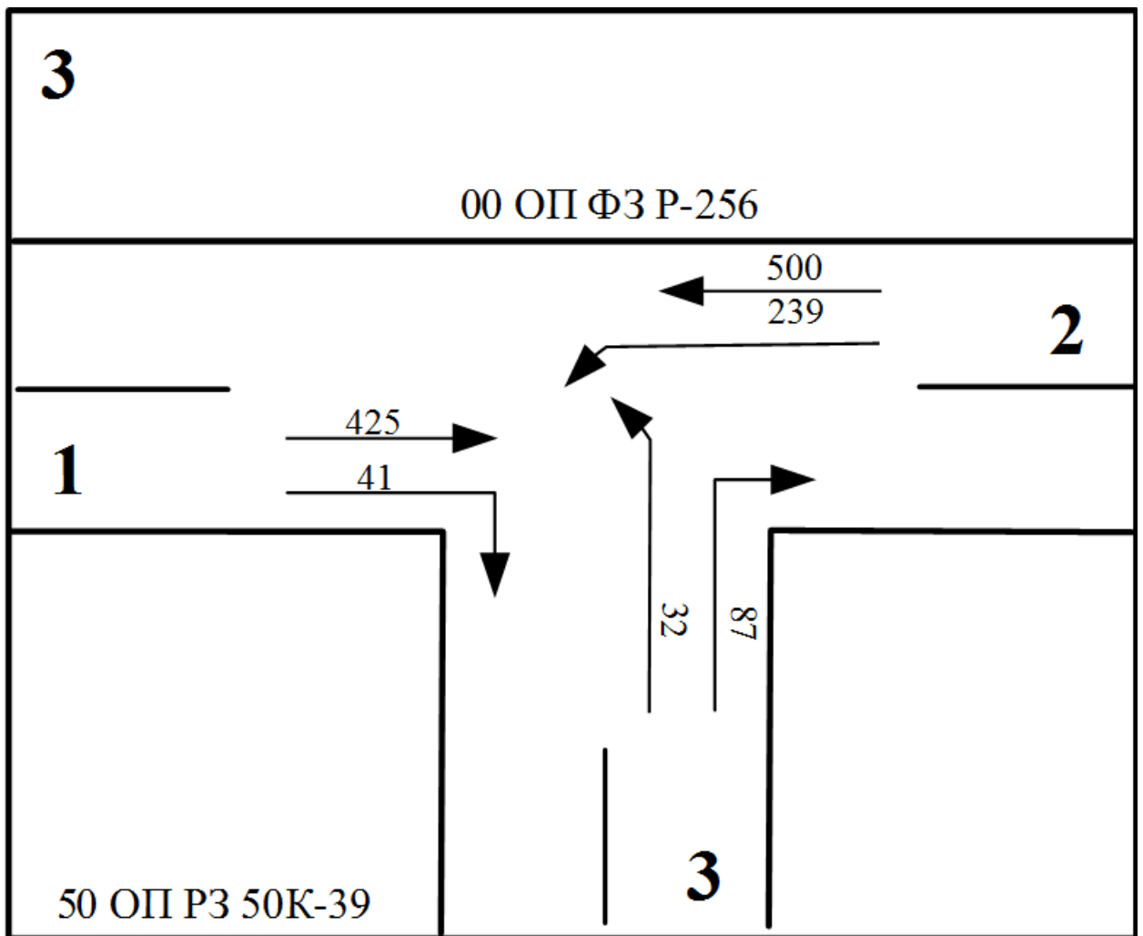
Рисунок 3 – Схема интенсивности движения ТС узла 3
