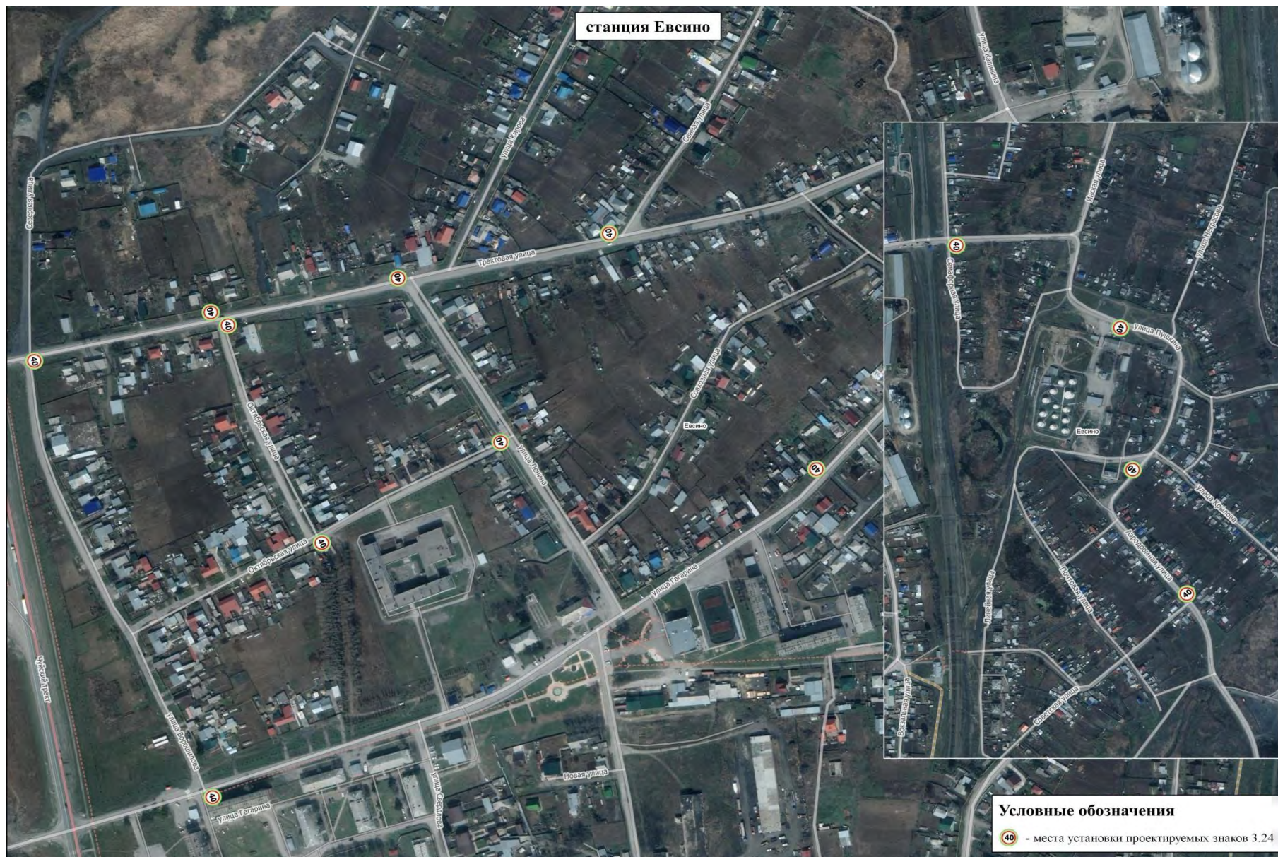
Рисунок 3.15.3 – Схема установки дополнительных знаков ограничения скорости
