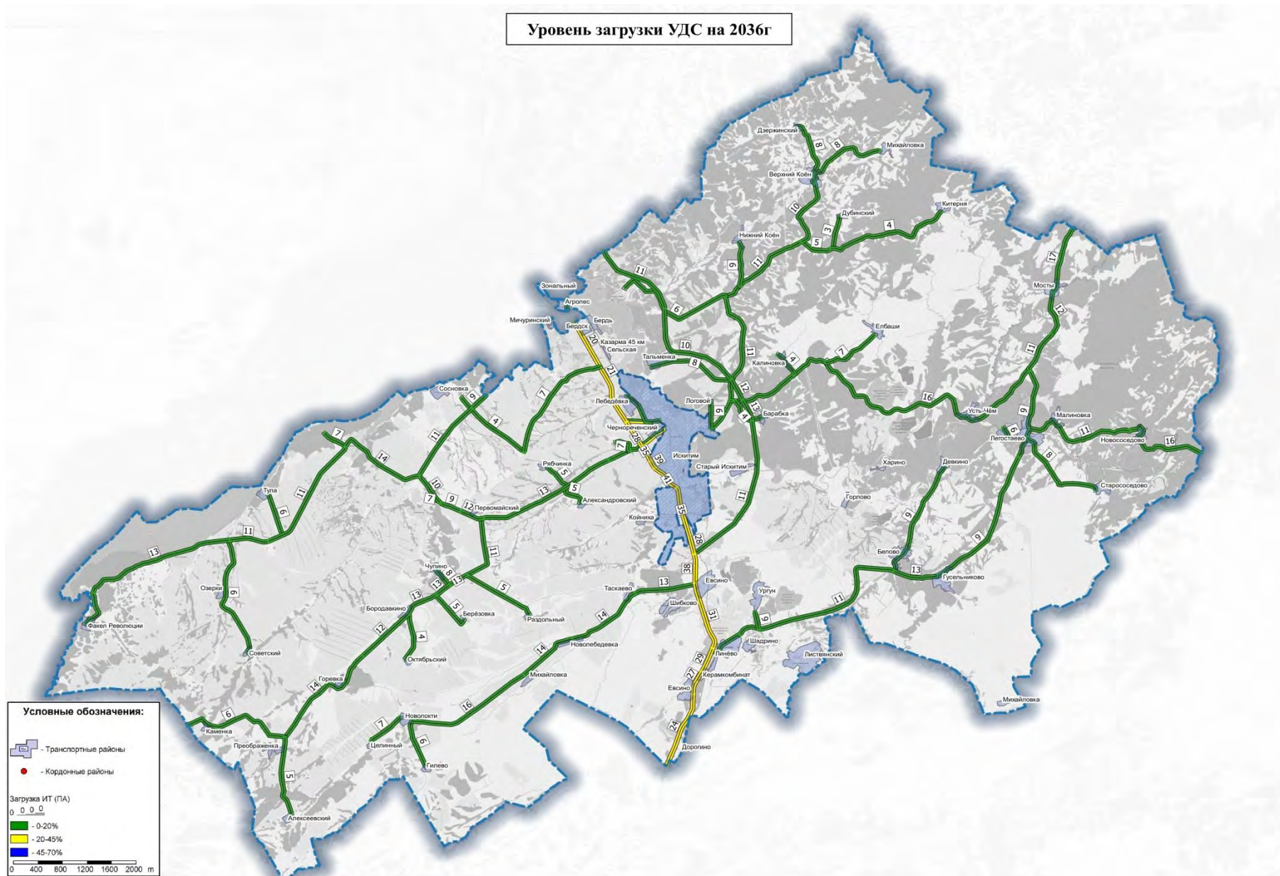
Рисунок 5.2 – Распределения уровней загрузки на 2036 год
