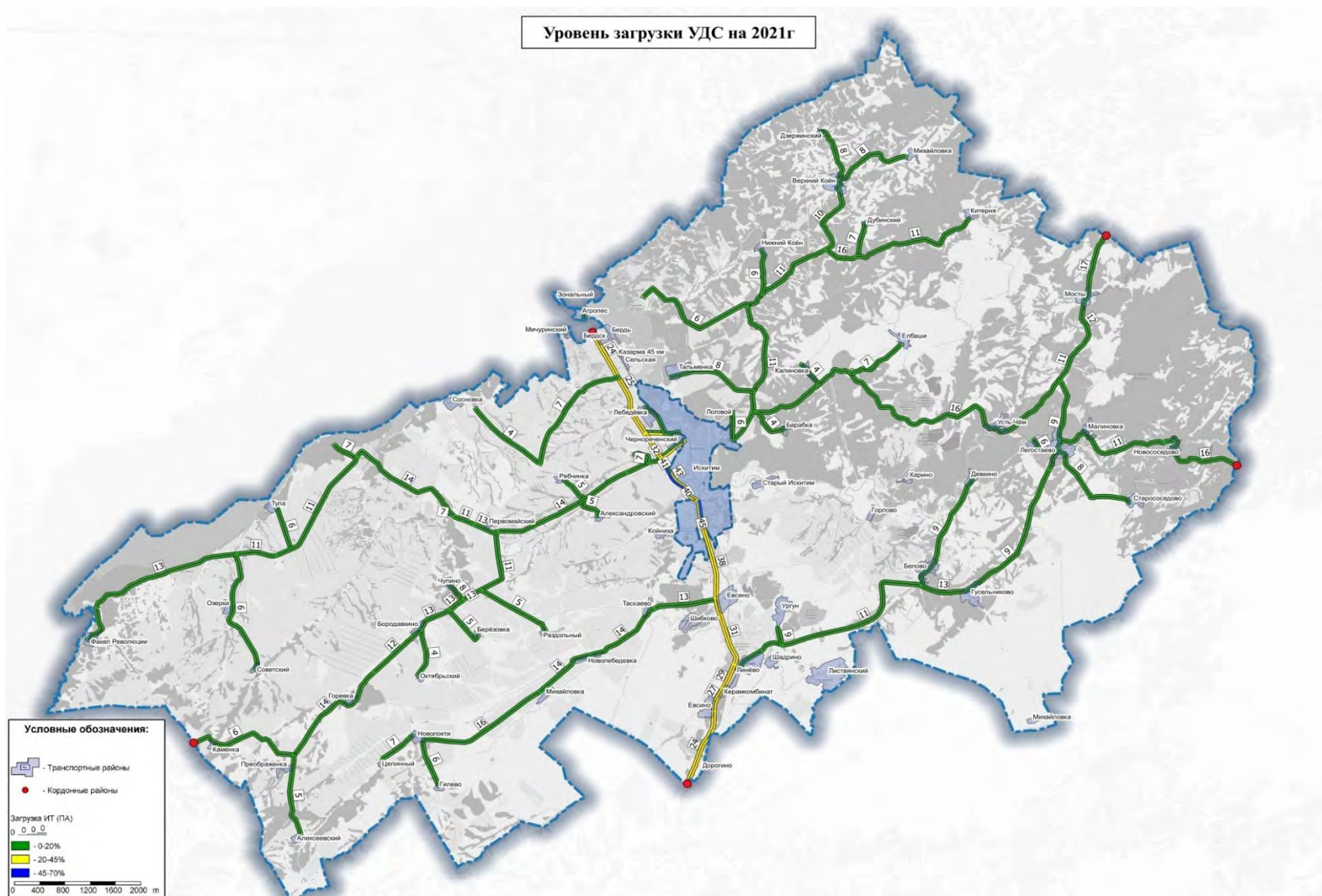
Рисунок 1.8.10 – Результаты расчета коэффициентов загрузки основных автомобильных дорог для существующей дорожно-транспортной ситуации
