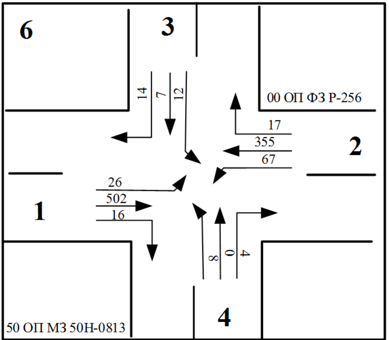
Рисунок 6 – Схема интенсивности движения ТС узла 6
