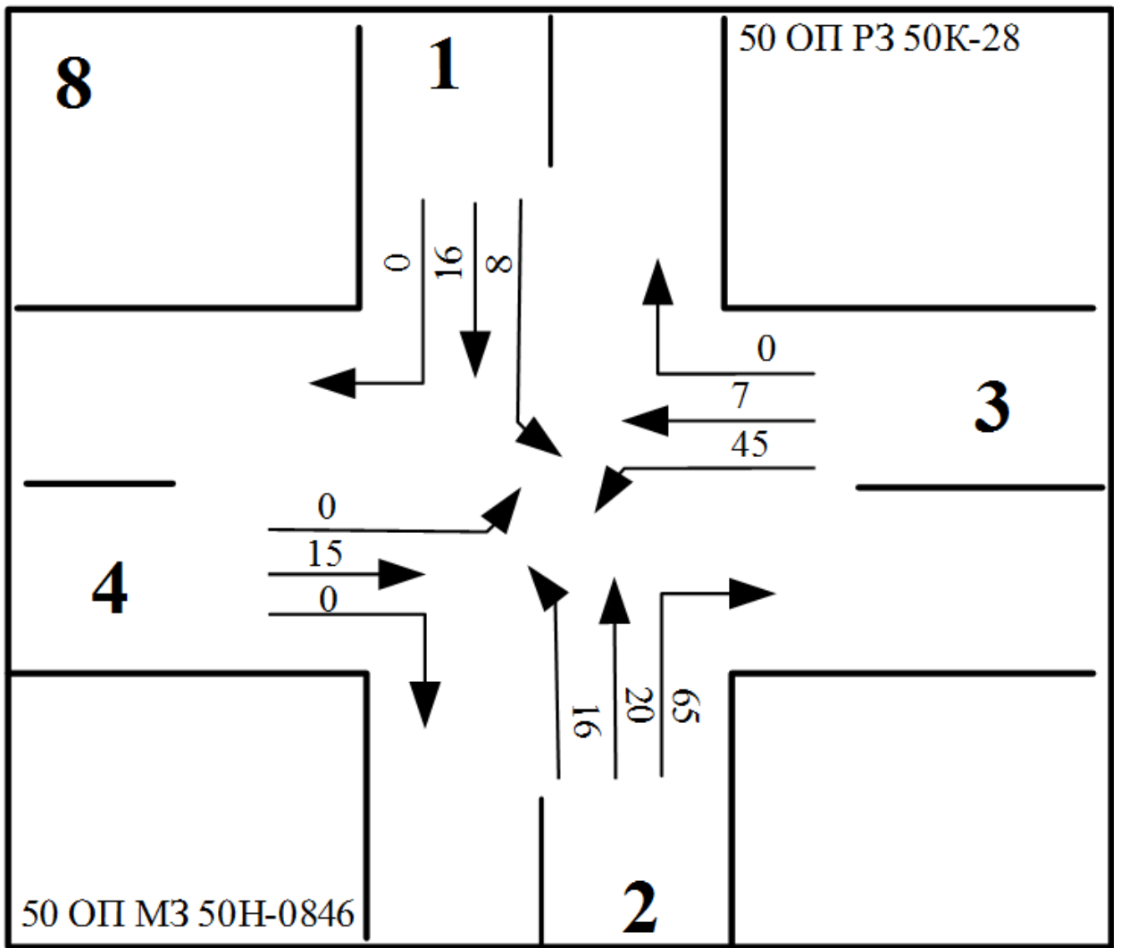
Рисунок 8 – Схема интенсивности движения ТС узла 8
