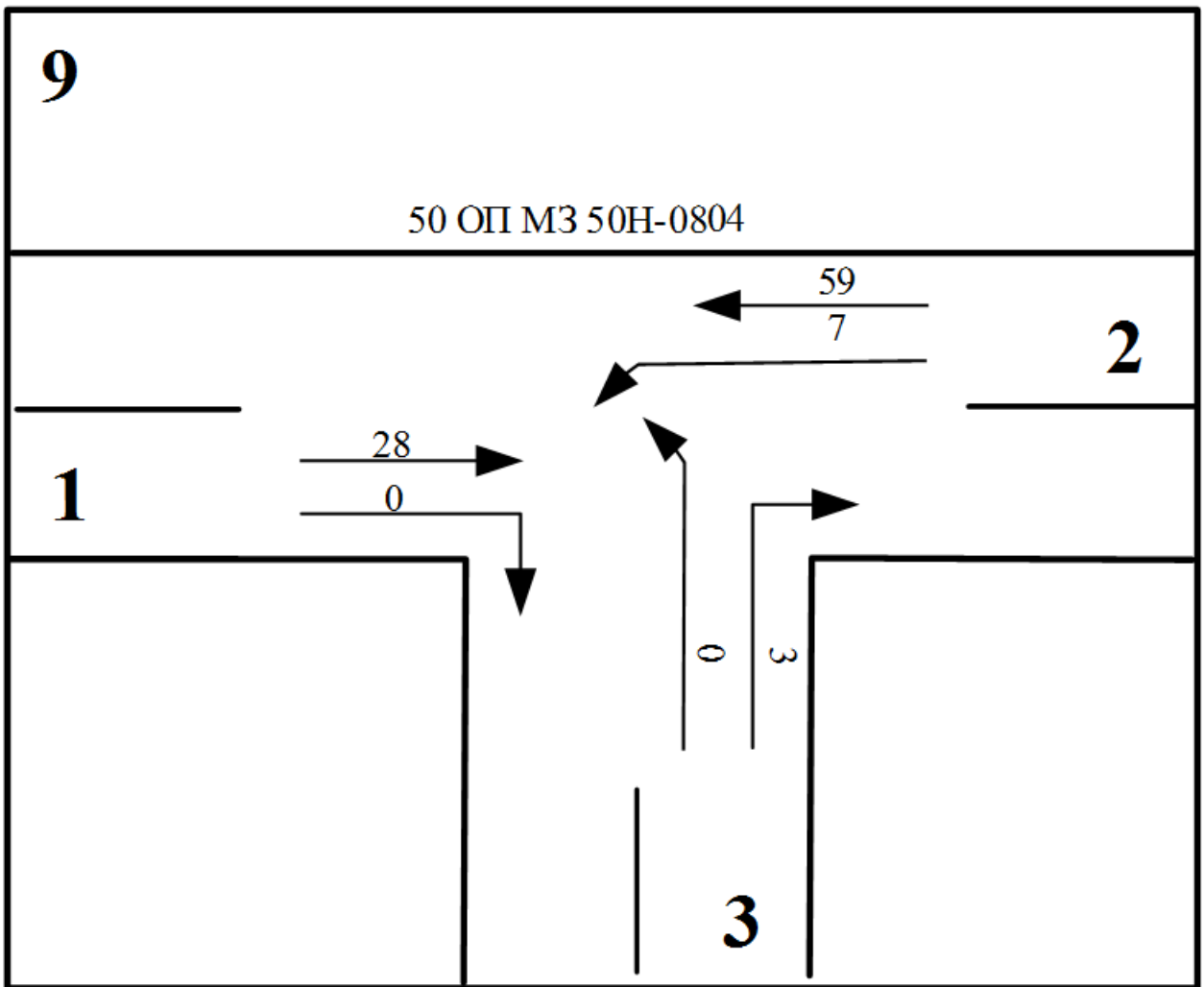
Рисунок 9 – Схема интенсивности движения ТС узла 9
