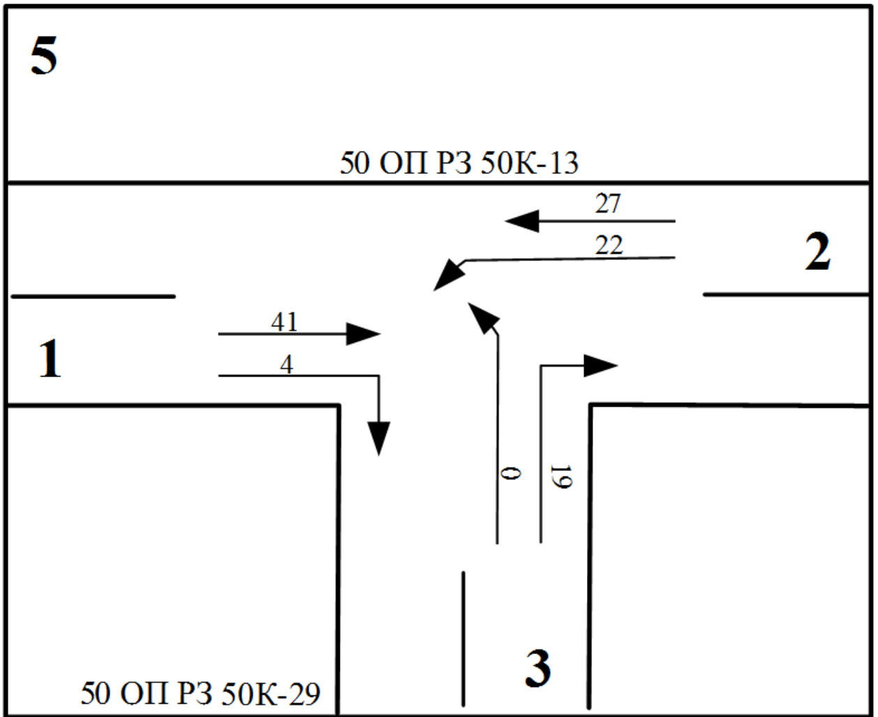
Рисунок 5 – Схема интенсивности движения ТС узла 5
