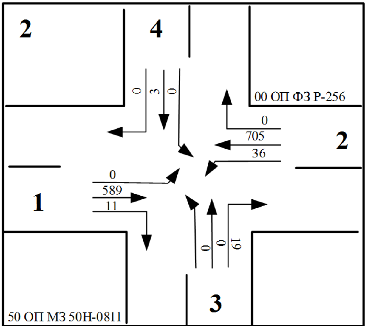
Рисунок 2 – Схема интенсивности движения ТС узла 2
