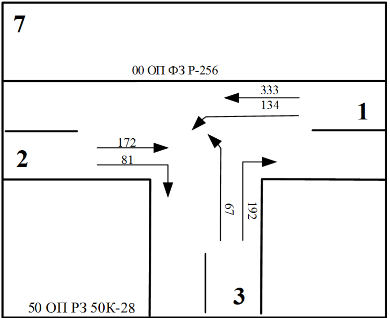
Рисунок 7 – Схема интенсивности движения ТС узла 7
